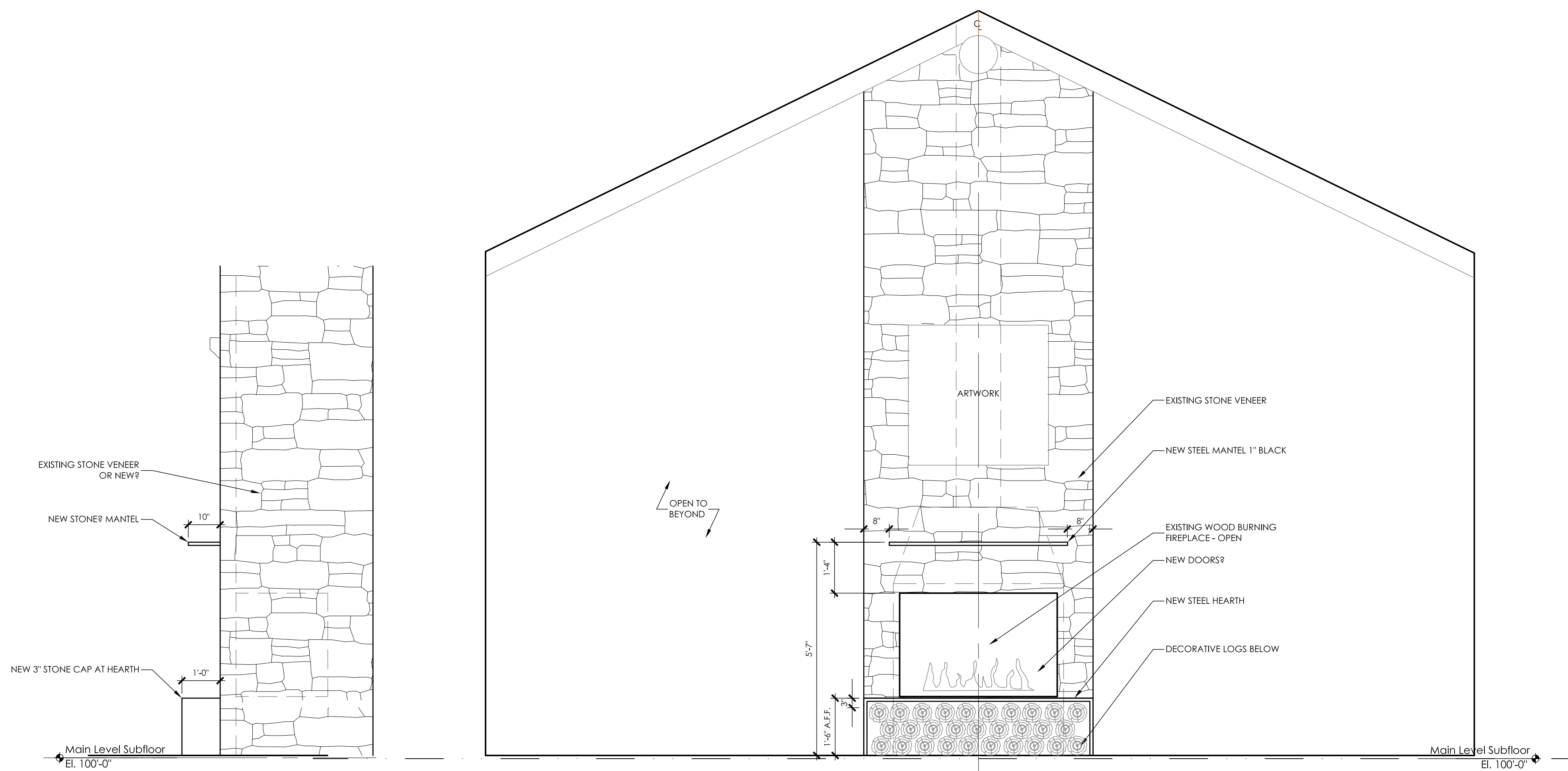
1 A3.2 FIREPLACE ELEVATION SCALE: 1/2" = 1'-0"
